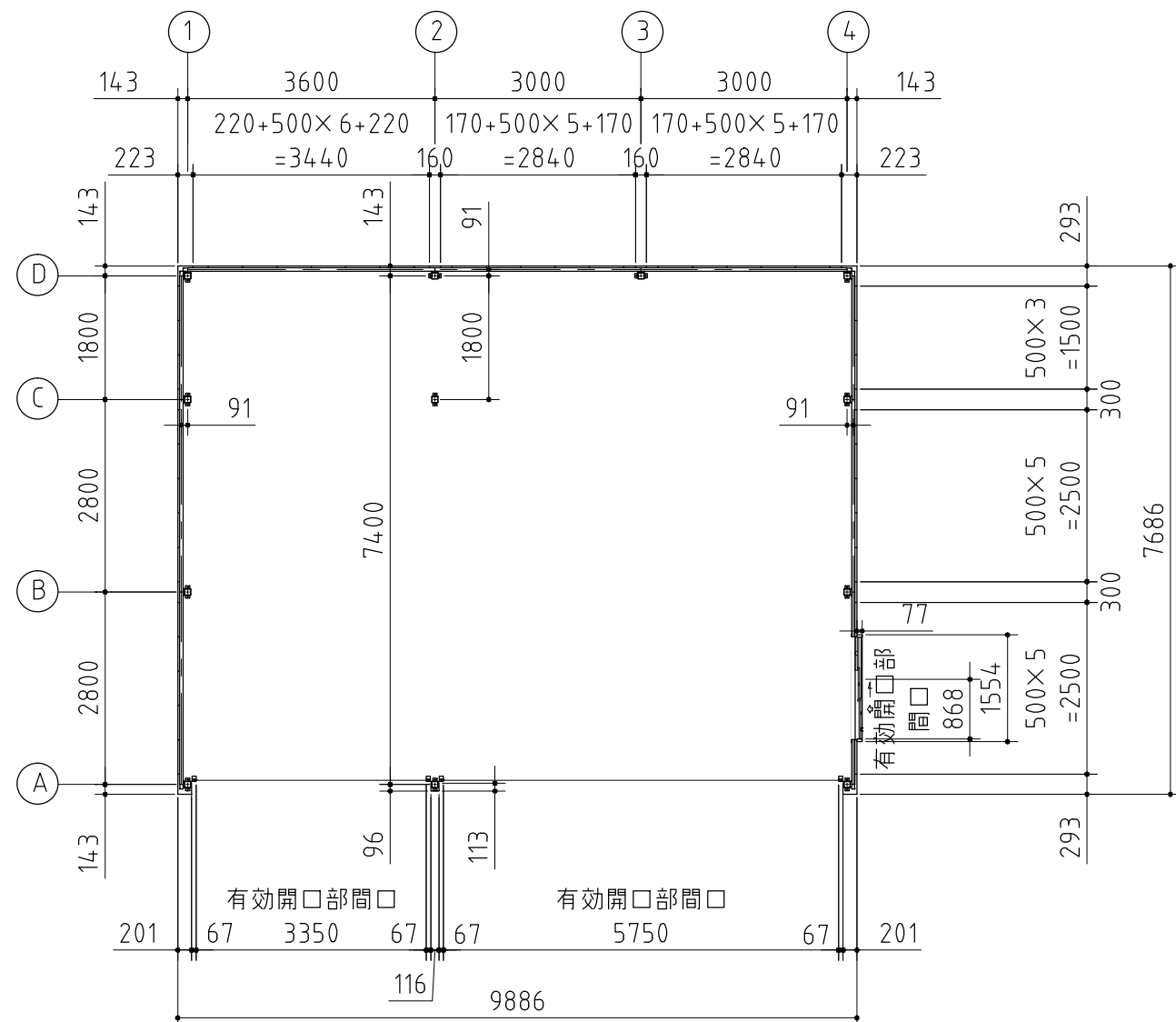
平面図
