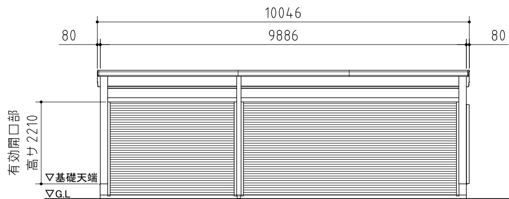
正面図
